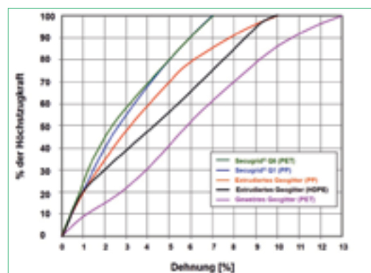
Abbildung 6: Zugkraft-Dehnungs-Kurven von Secugrid® und ausgewählten Geogittern
