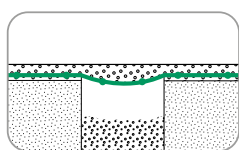
Abbildung 5: Überbrückung von Erdfällen und Tages- brüchen
