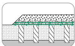
Abbildung 4: Lastverteilungspolster über vertikalen Tragelementen
