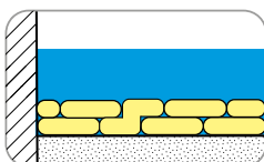
Abbildung 3: Kolkschutz
