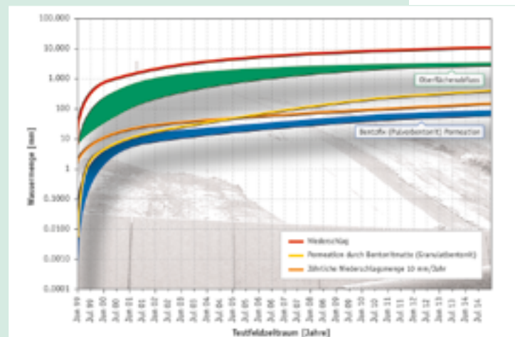
Abbildung 3 Niederschlag, Drainagewasserabfluss und Wasserpermeation durch geosynthetische Tondichtungsbahnen unter einer Bodenauflast von 1 m in deutschen Klimaverhältnissen
